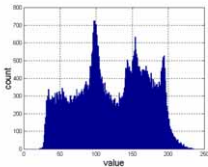
分布
