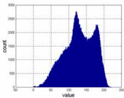
分布
