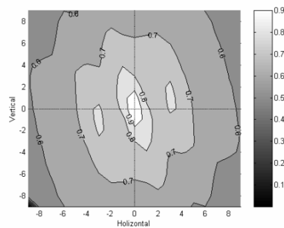
相関係数
