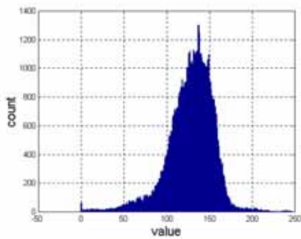
分布
