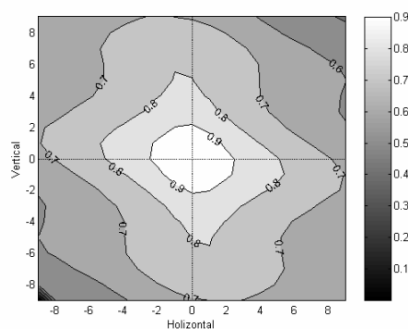
相関係数
