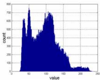
分布
