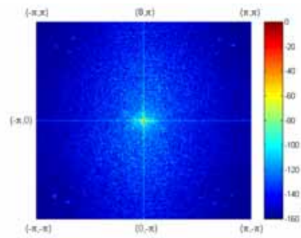
相関係数
