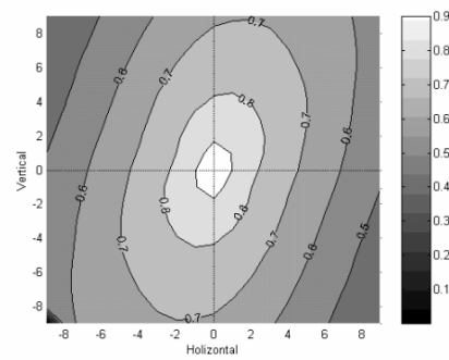
相関係数
