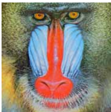
分布
